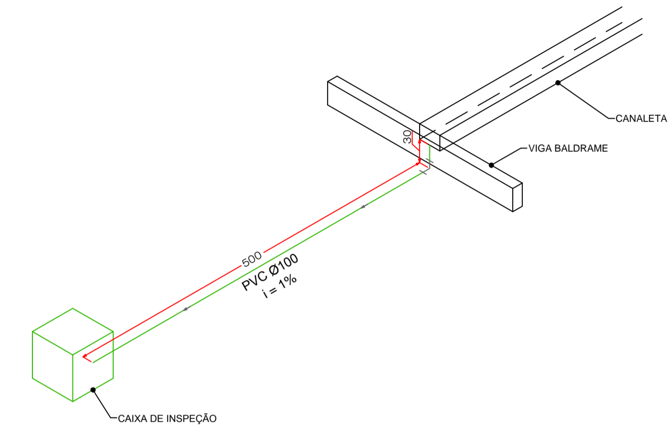
DETALHE DA TUBULAÇÃO Esc 1:100
