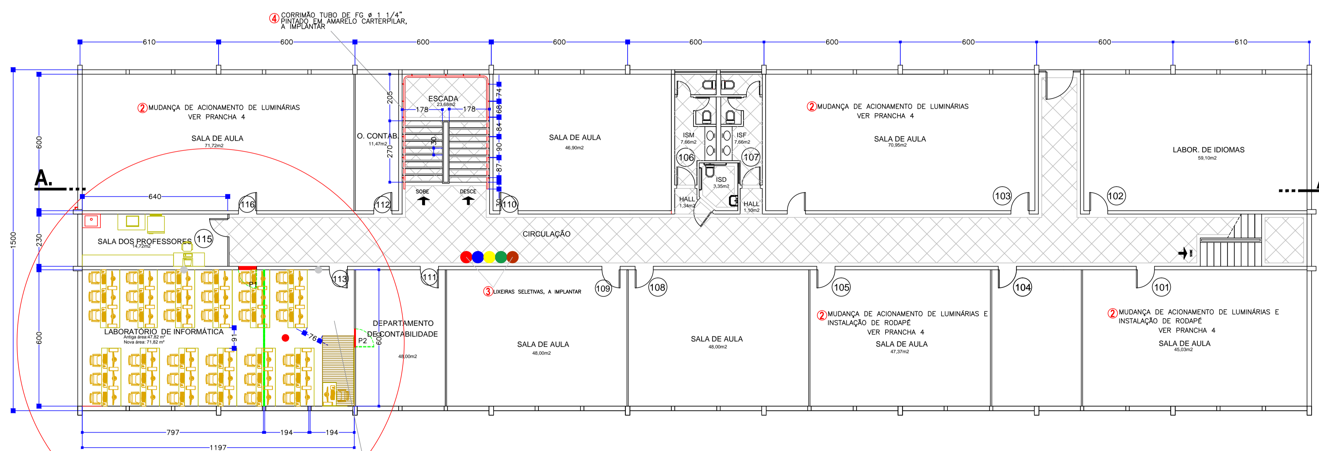
PLANTA DO NÍVEL 2 - 2º PAVIMENTO
