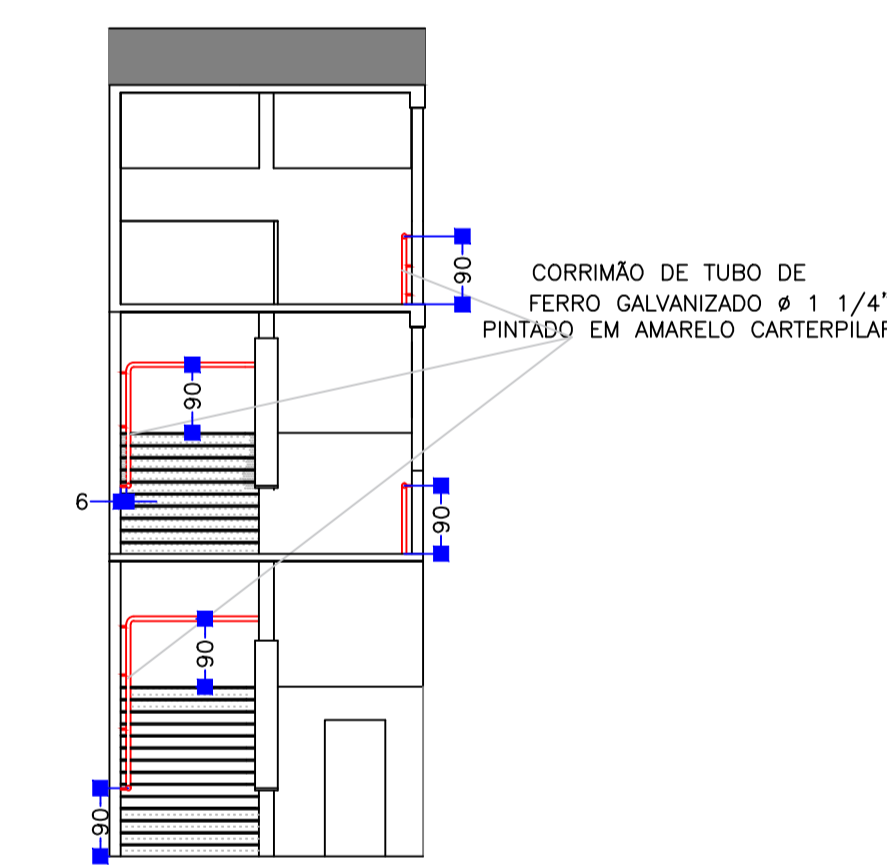
DETALHE: CORRIMÃO (corte A-A)
