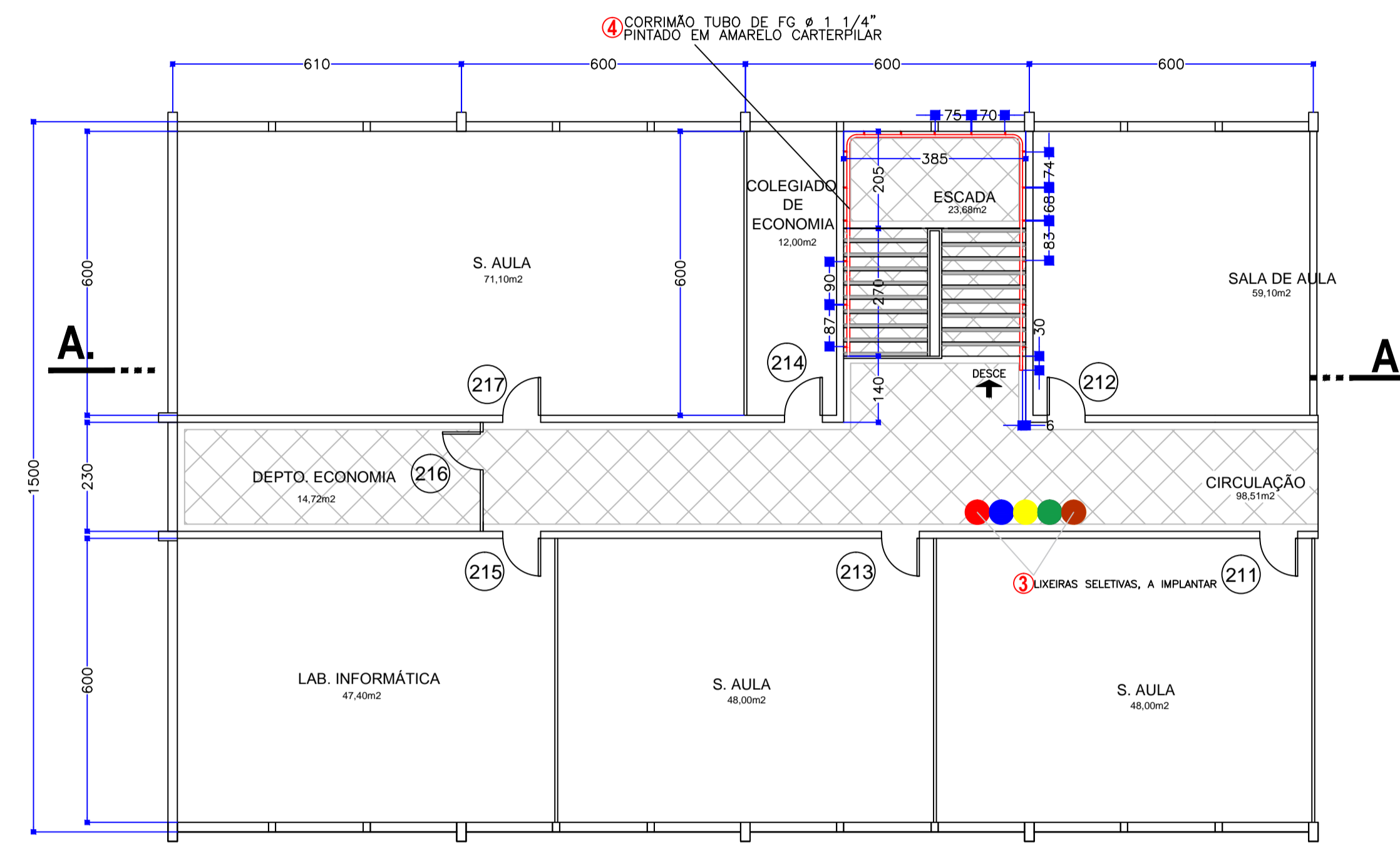
PLANTA DO NÍVEL 3 - 3º PAVIMENTO
